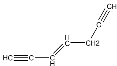
3-hepten-1,6-diino
