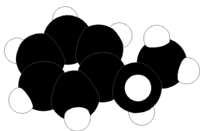
1-etil-3-metilbentzenoa
