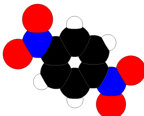
1,3-ziklohexadienoa
