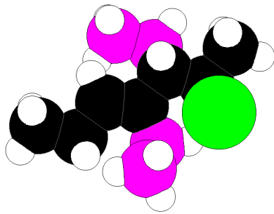
5-kloro-4,4-dimetil-2-heptinoa
