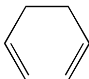
1,3-ziklohexadienoa
