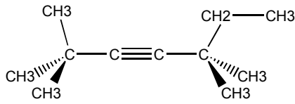
2,2,5,5-tetrametil-3-heptino
