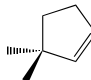
3,3-dimetilziklopentenoa
