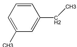
1-etil-3-metilbentzenoa
